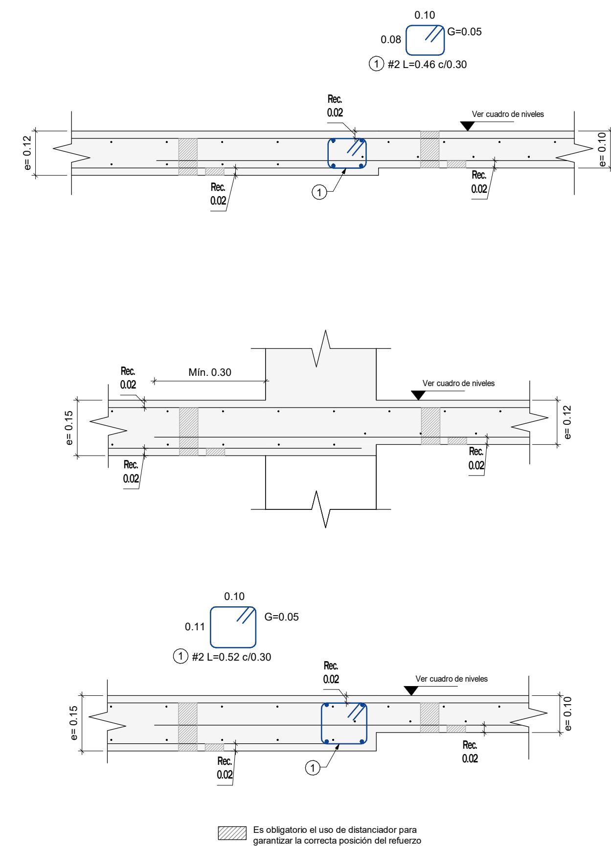
DETALLES TÍPICOS - CAMBIO DE SECCIÓN Escala 1 : 10
