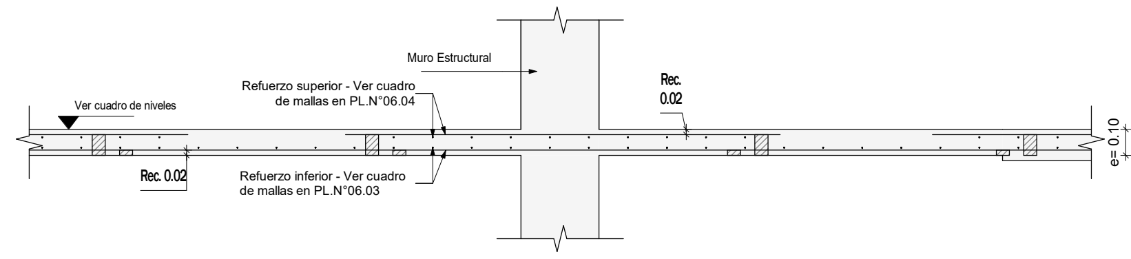
CORTE TÍPICO PLACA AÉREA e=0.10 Escala 1 : 20
