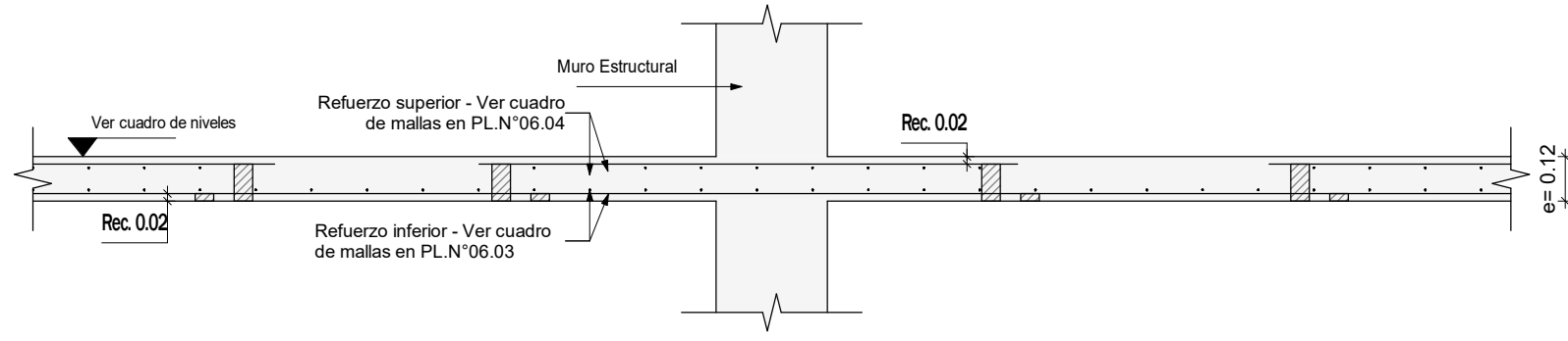
CORTE TÍPICO PLACA AÉREA e=0.12 Escala 1 : 20
