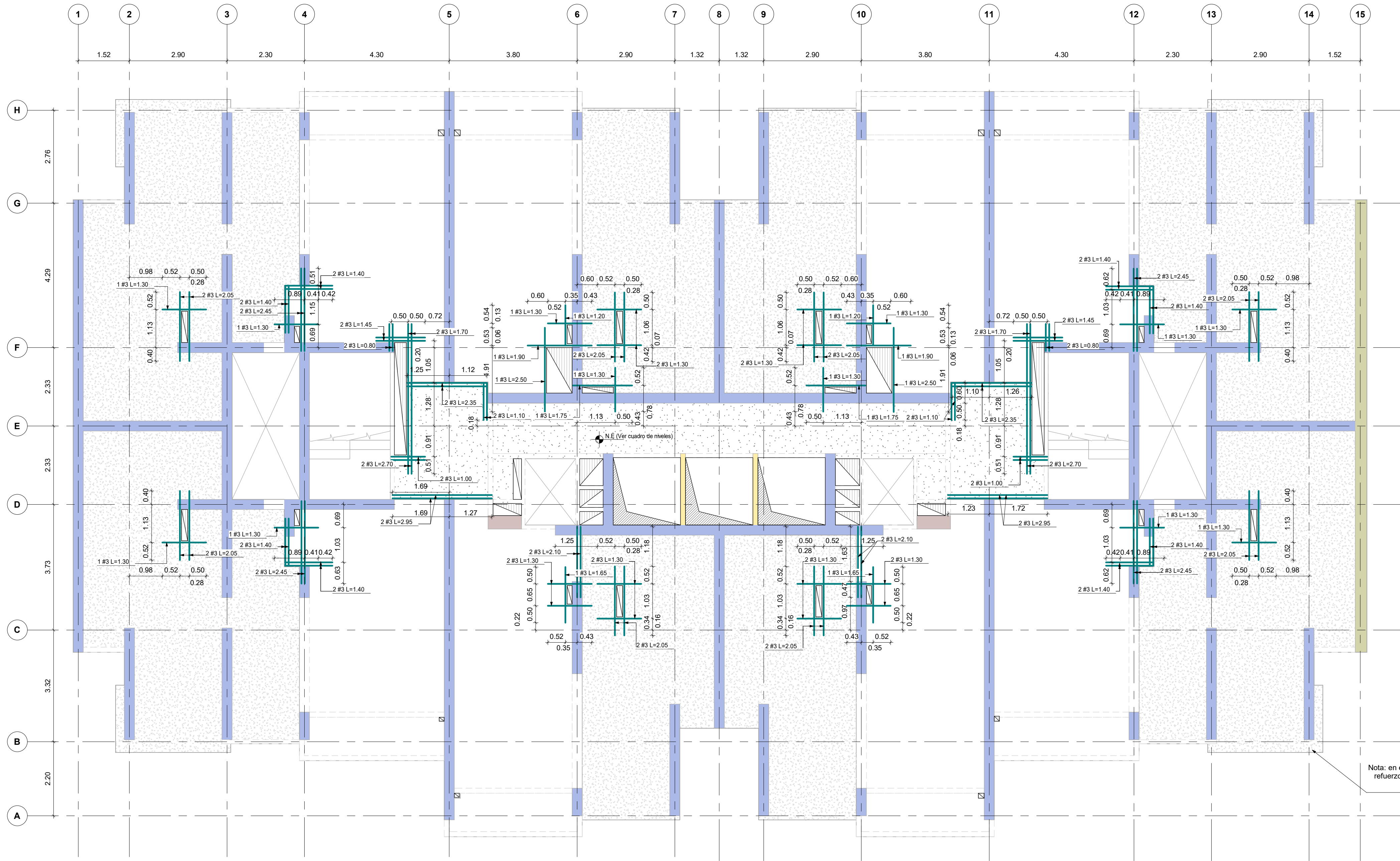
PLANTA DE REFUERZO ADICIONAL PISO TIPO 1 ( PISO 3 A PISO 15 ) Escala 1 : 75
