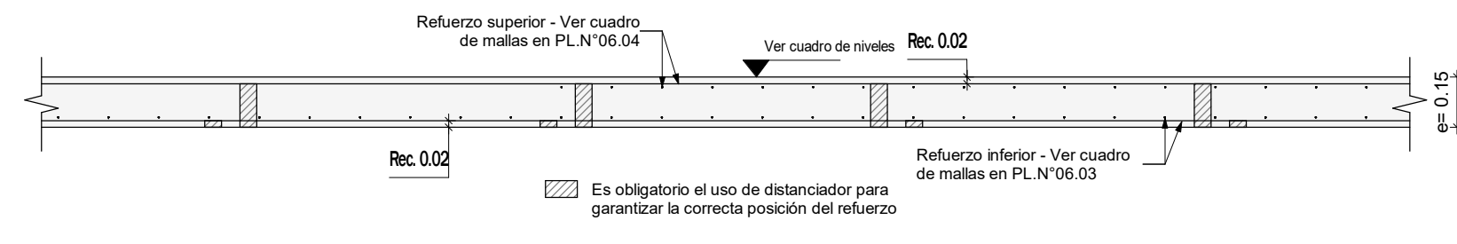
CORTE PLACA AÉREA e=0.15 Escala 1 : 20
